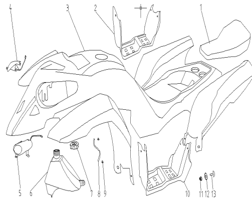
7 FENDER 覆盖件
