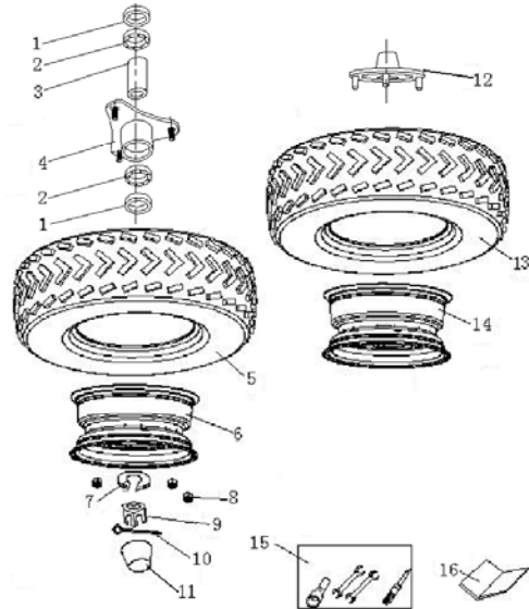
6 TYRE 轮系
