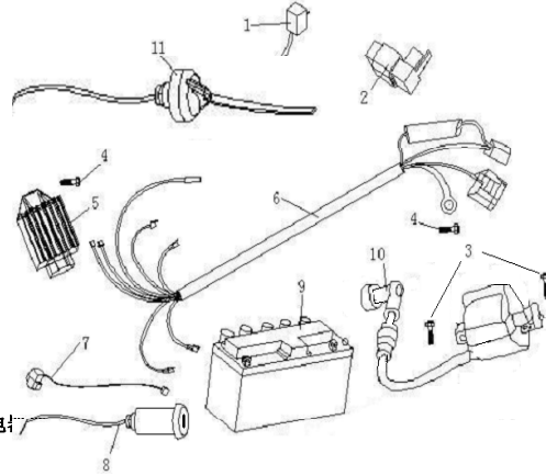
5 ELECTRIC HARDBESS 电
